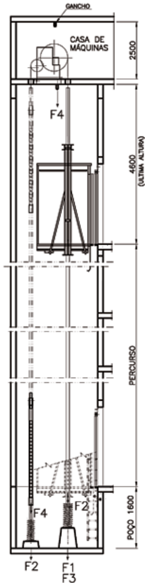
Corte Esquemático
