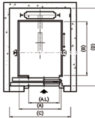
Planta Baixa
